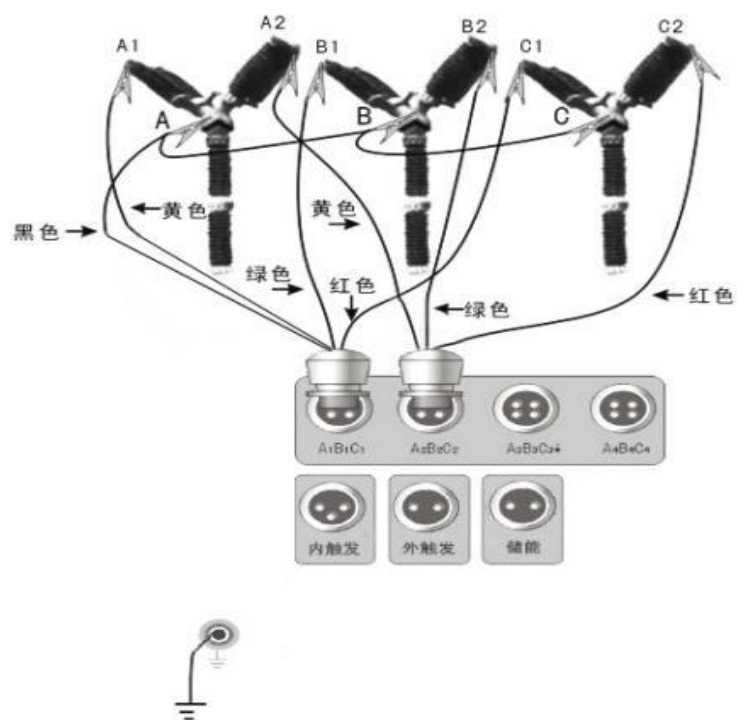
断口接线图（六断口）
